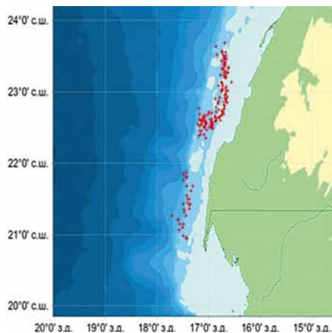
Рисунок 1. Места сбора данных в ЦВА с 2004 по 2017 годы
